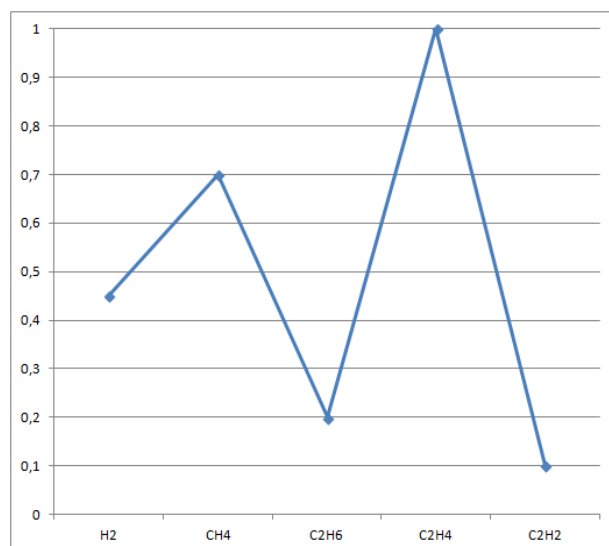
б) Образ дефекта - высокотемпературный нагрев
