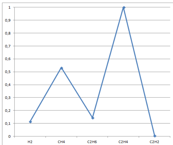
а) Диаграмма АРГ трансформатора
