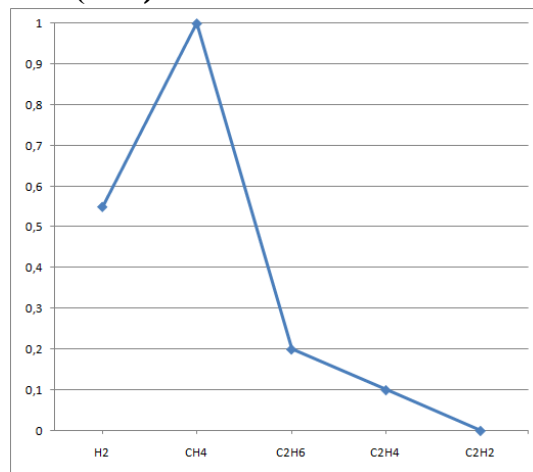
Рис. 8. Нагрев, сопровождающийся ЧР
