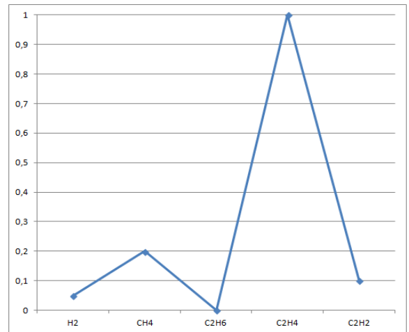
б) Образ дефекта - нагрев в диапазоне средних температур
