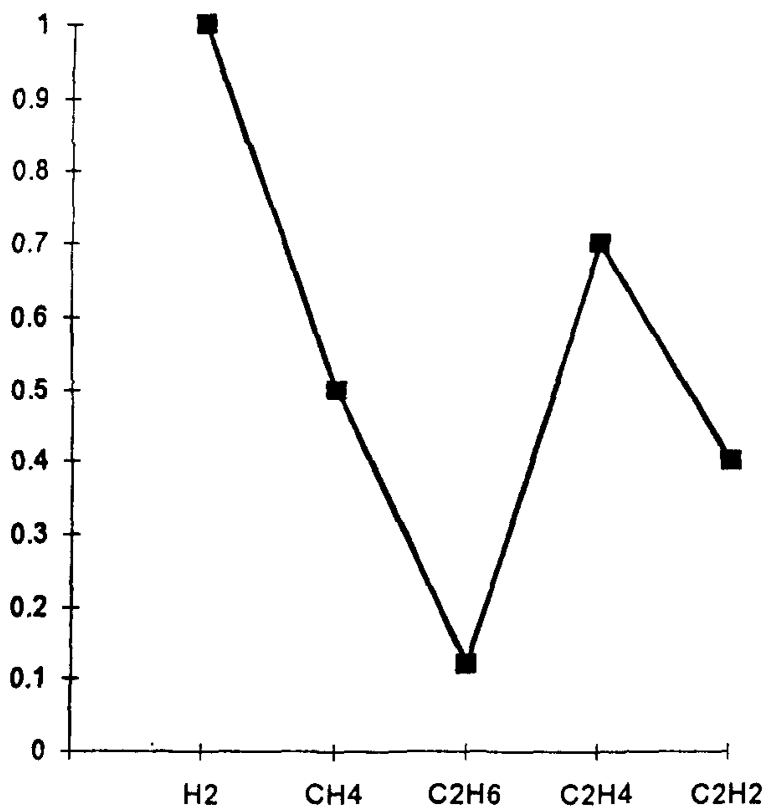
Рис. 3.3. Дефекты, вызванные искрением
