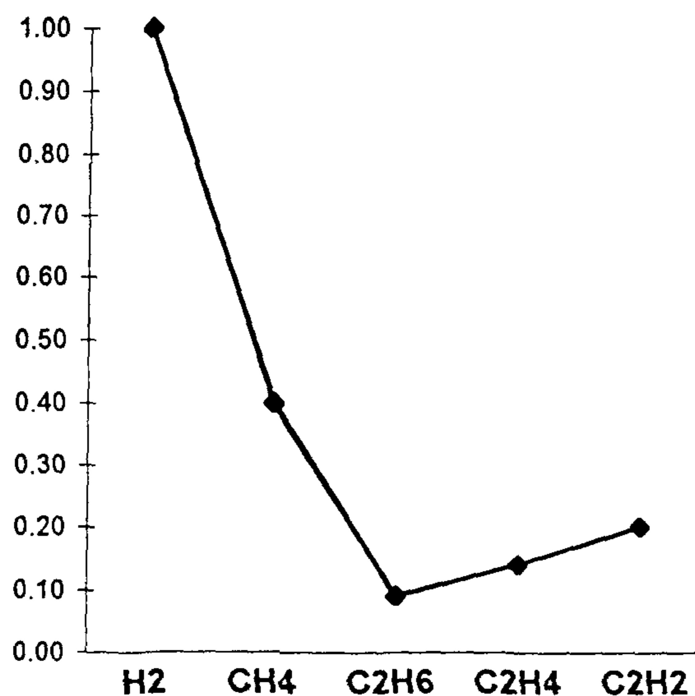
Рис.3.1. Разряды малой мощности
