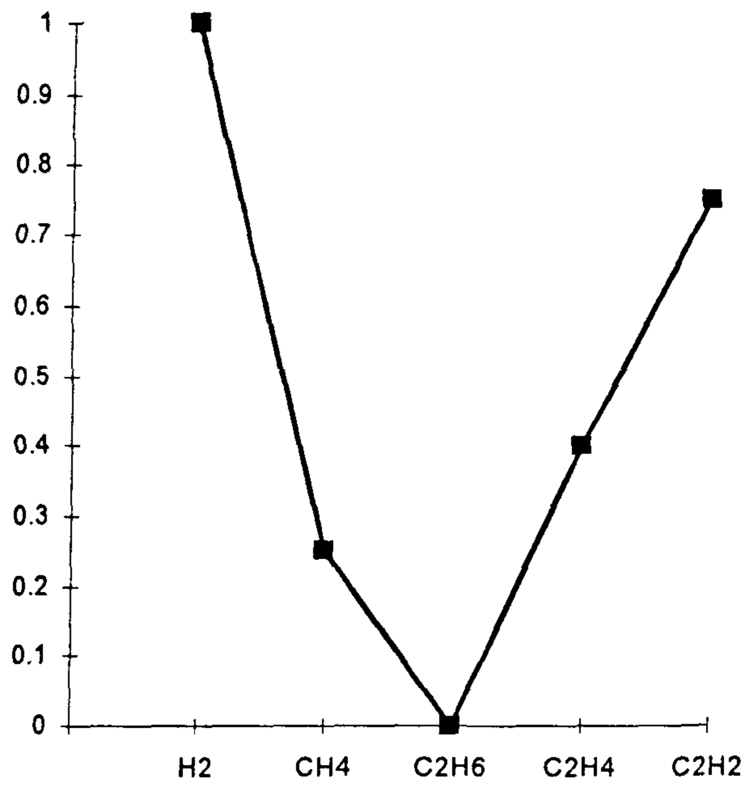
Рис. 3.4. Дефекты, вызванные дугой
